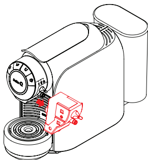
Rys. 32: Odłączyć system dozowania mleka.
