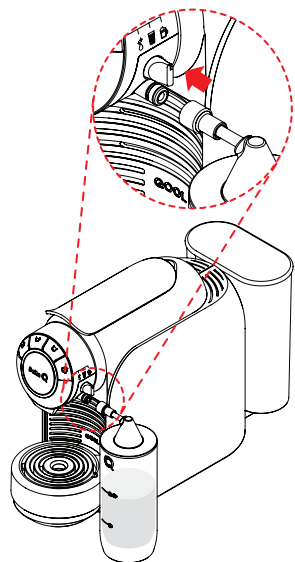
Fig. 20: Conectar o depósito de leite ao sistema de leite.
