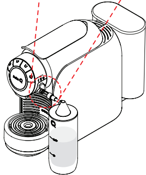
Fig. 20: Conecte el depósito de leche al sistema de leche.
