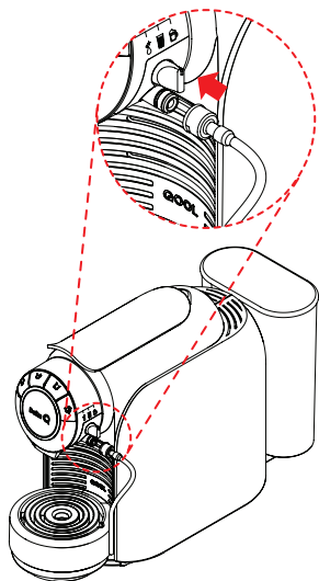
Rys. 23: Podłączyć rurkę ssącą do systemu dozowania mleka.
